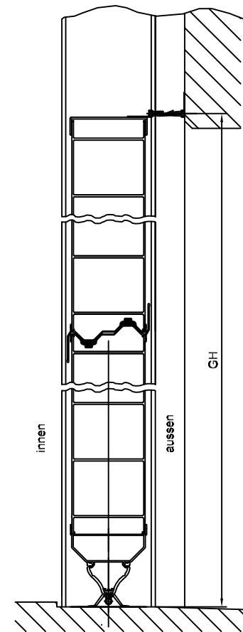
Vertikalschnitt
